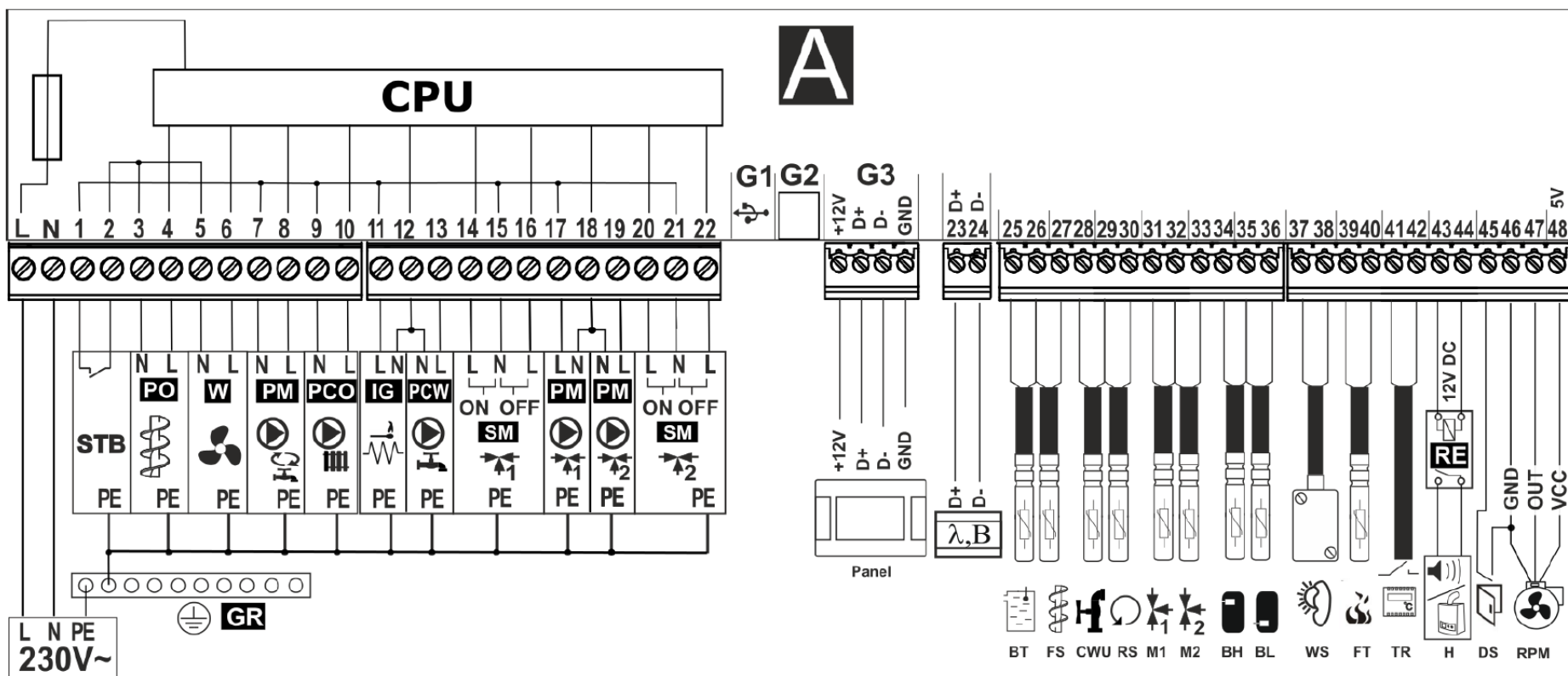
Rysunek 17.1 Schemat elektryczny podłączenia kotła – sterownik PLATINUM.
