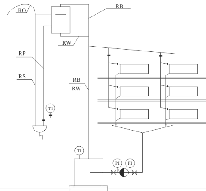
Rysunek 1514.1 Schemat podłączenia kotła do instalacji grzewczej
