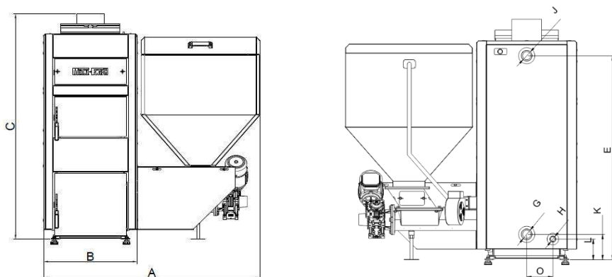
Rysunek9.1 Wymiary kotła SMART EKO-CARBON
