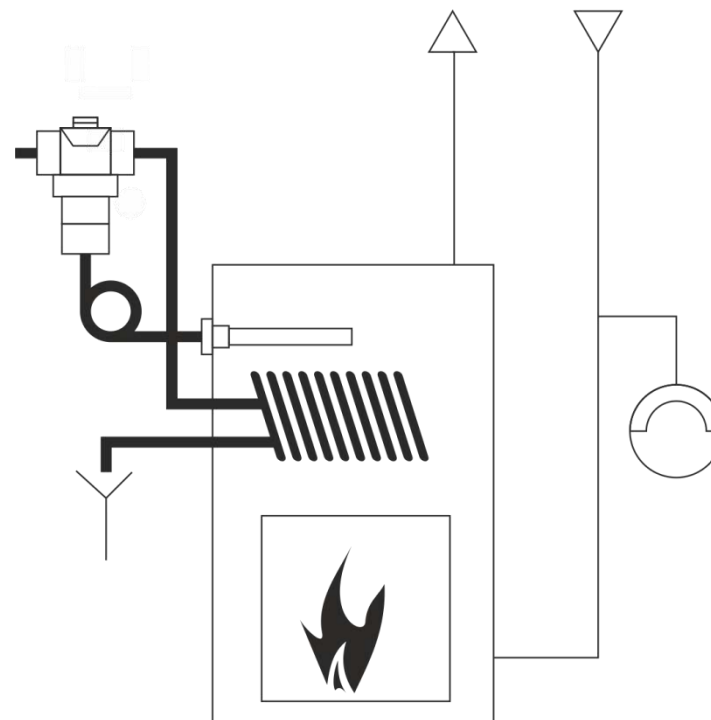
Rysunek 15.1 Schemat zabezpieczenia kotła za pomocą wbudowanej wężownicy chłodzącej i z zabezpieczeniem termicznym.
