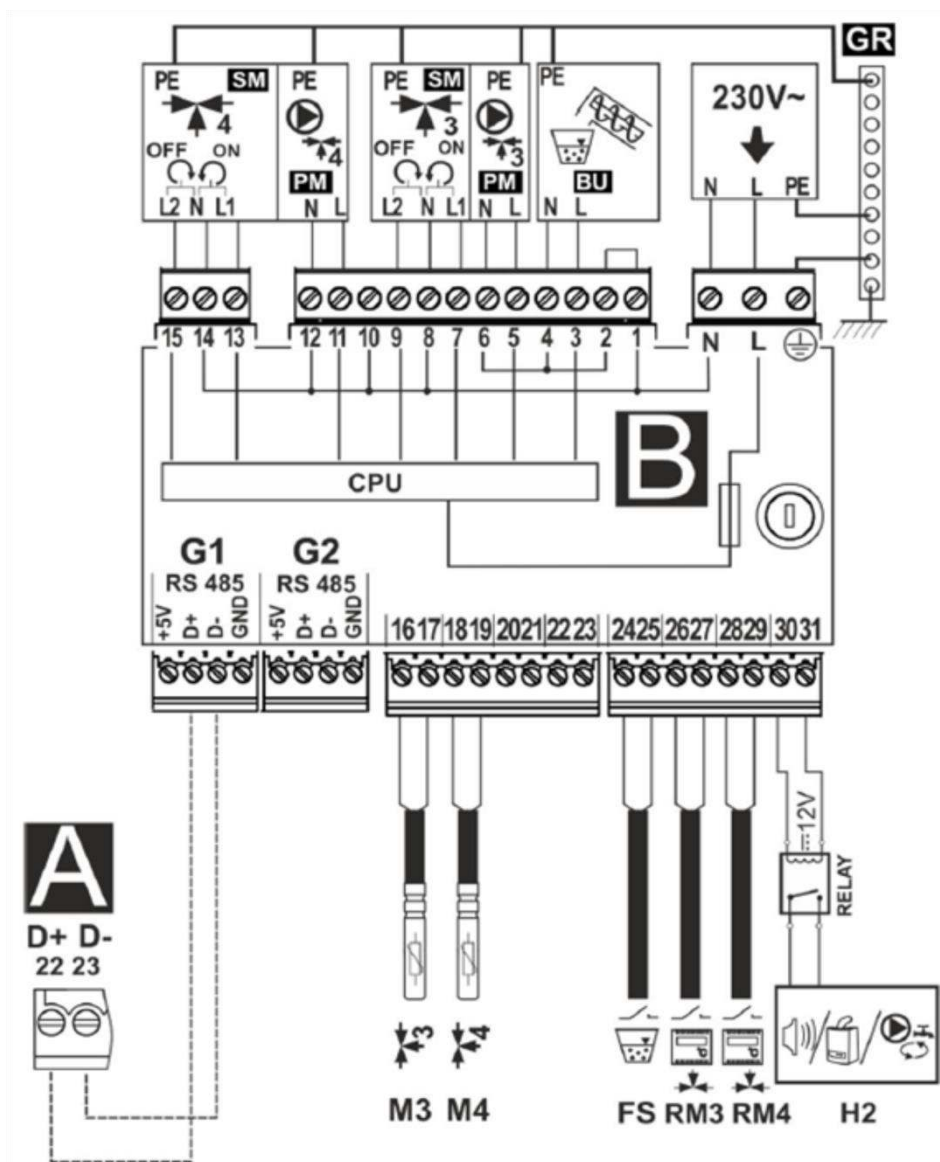
Rysunek 177.2 Schemat elektryczny podłączenia kotła.
