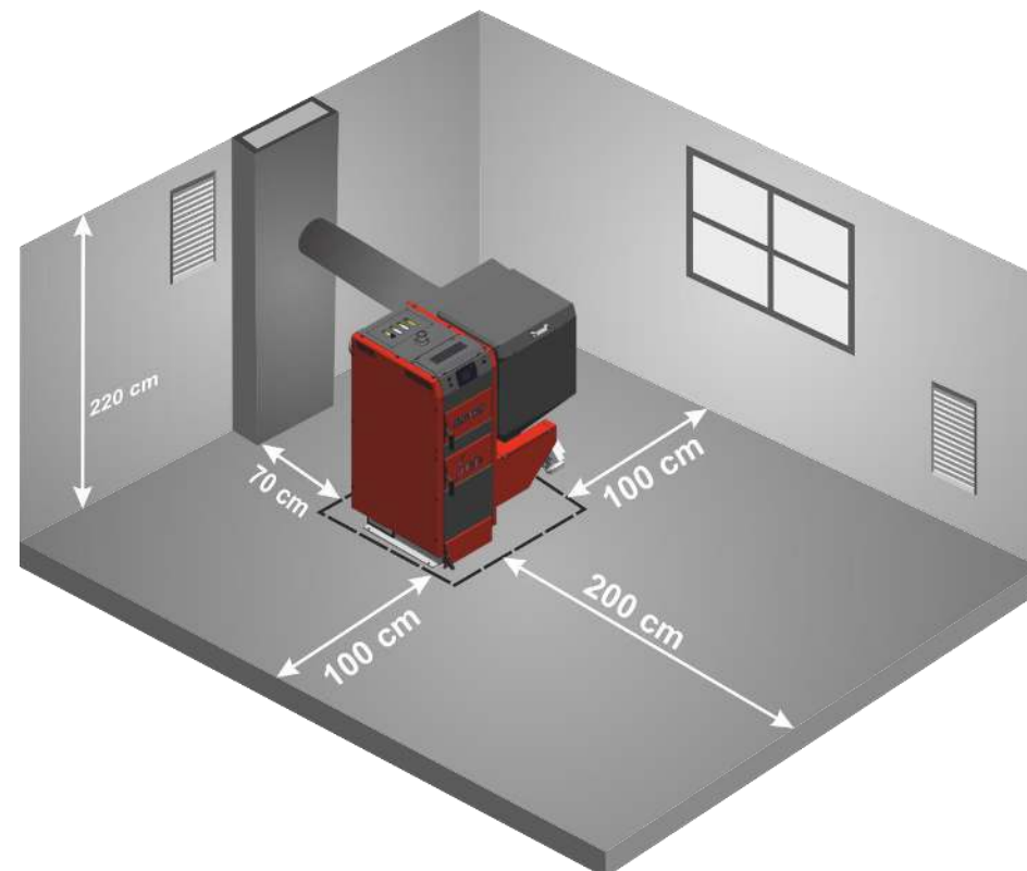
Rysunek 13.1 Minimalne odległości ustawienia kotła w kotłowni
