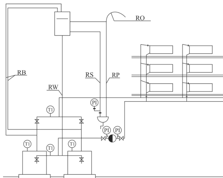
Rysunek 15.2 Schemat podłączenia kotła do instalacji grzewczej
