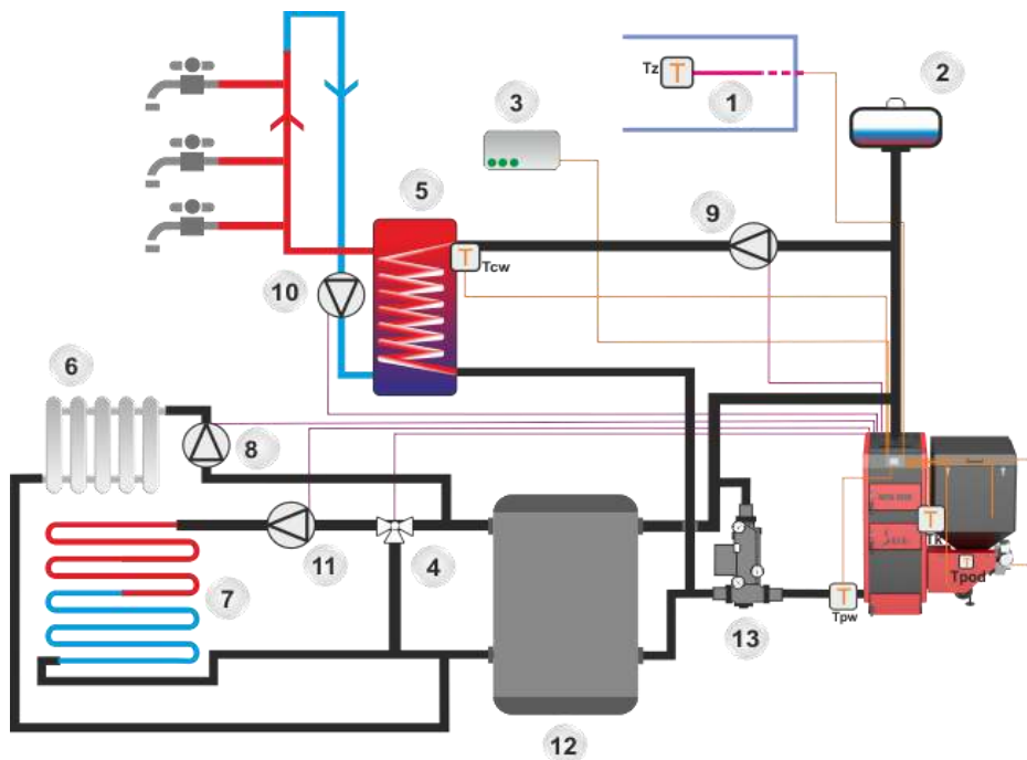
Rysunek 15.4 Podłączenie kotła do instalacji grzewczej z laddomatem i buforem
