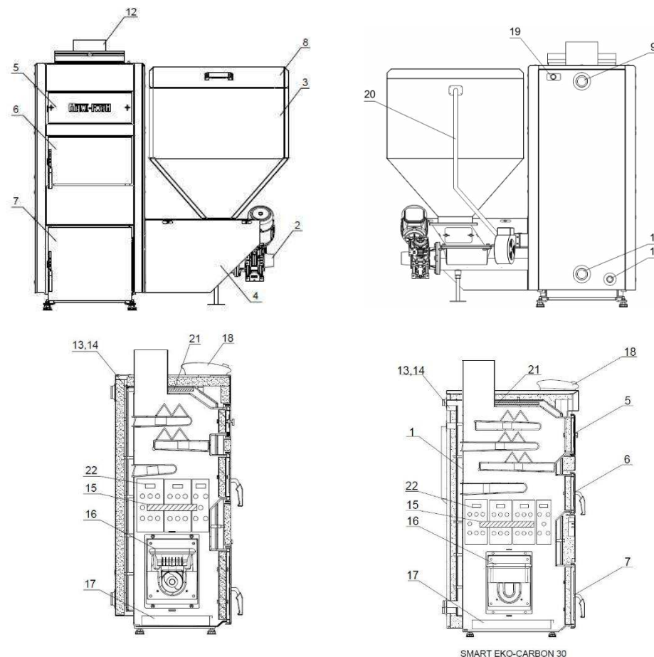
Rysunek 7.1 Podstawowe elementy budowy kotła SMART EKO-CARBON
