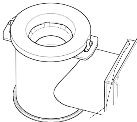
KROK 5. Poprawnie zmontowany palnik retortowy z wycelowaną płytą i koroną paleniska
