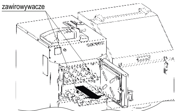
KROK 4. Ostrożnie wysunąć zawirówywasze. Oczyszczyć zawirówywasze oraz powierzchnię wymiany ciepła. Zamontować w odwrotnej kolejności
