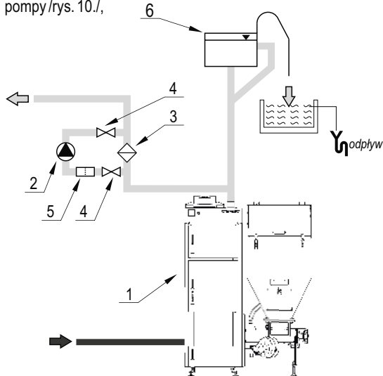
Rysunek 10. Wykonanie obejścia grawitacyjnego: 1-kocioł; 2-pompa obiegowa; 3-zawór różnicowy; 4-zawory odcinające; 5-filtr; 6-otwarte naczynie zbiorcze.
