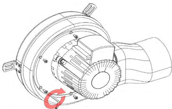
KROK 1. Odkręcić śruby mocujące wirnik wentylatora.
