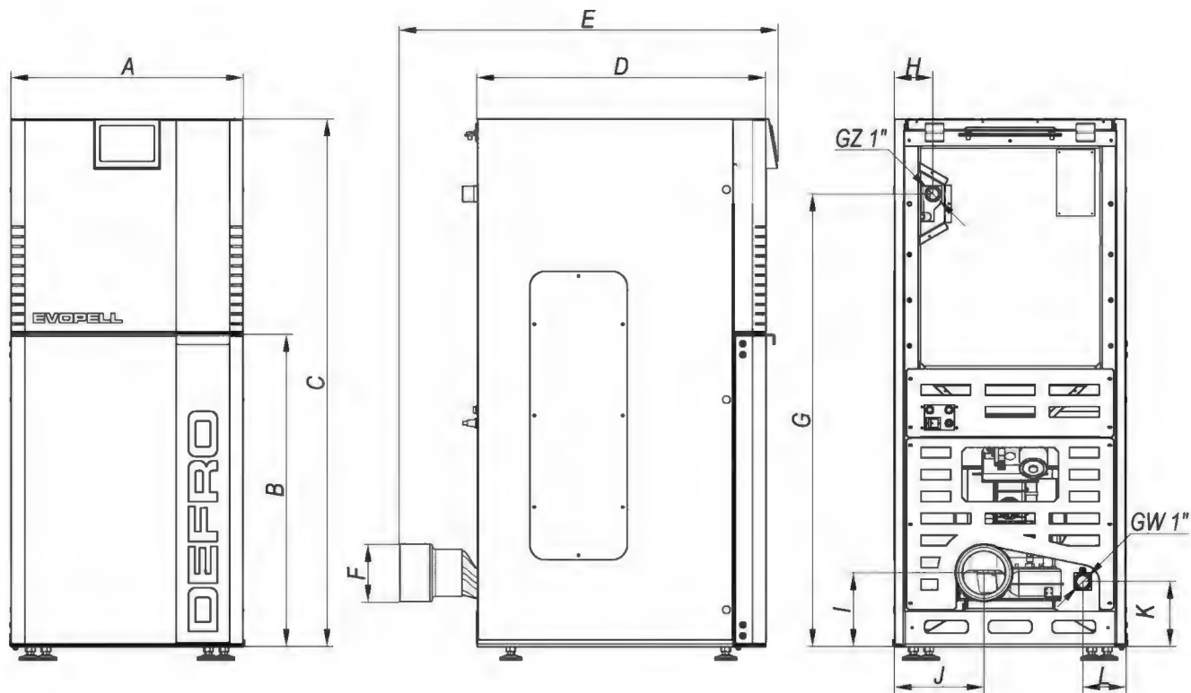
Rysunek 1. Podstawowe wymiary kotła.
