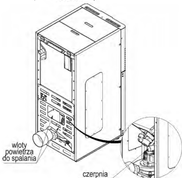
Rysunek 10. Czerpnia powietrza - otwór dolotowy powietrza.
