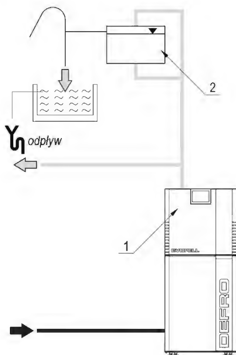
Rysunek 4. Przykładowy schemat zabezpieczeń kotła EVOPELL w układzie otwartym
