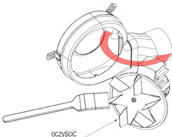
KROK 2. Oczyścić łopatki wirnika wentylatora.
