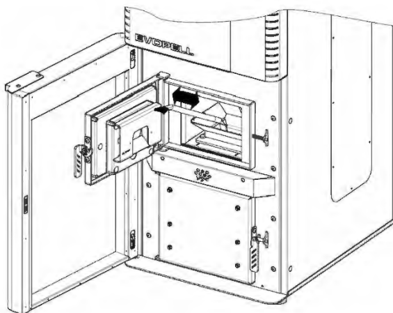
Rysunek 11. Sposób czyszczenia paleniska pelletowego.
