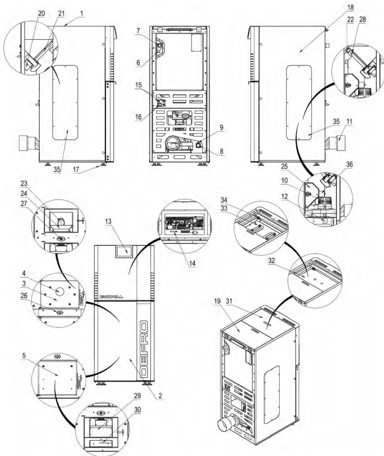
Rysunek 2. Podstawowe elementy kotła.
