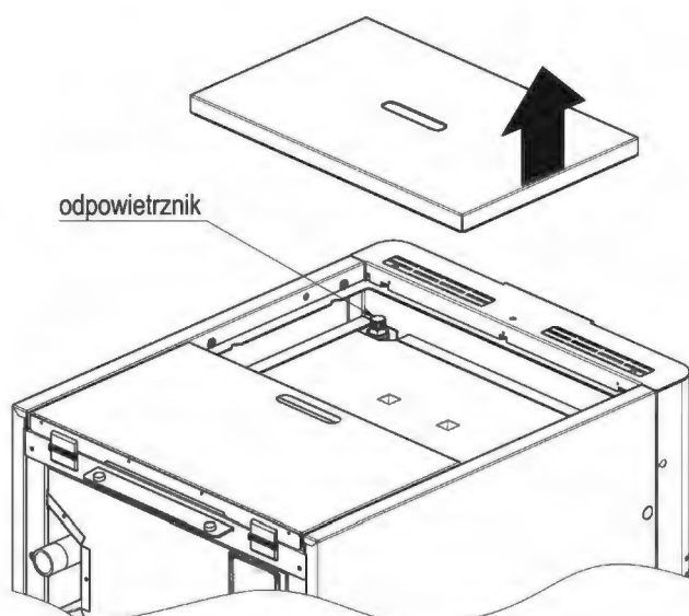
Rysunek 6. Odpowietrznik kotła.
