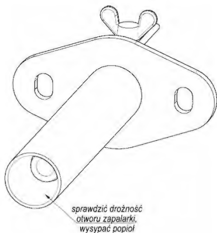
Rysunek 15. Sposób czyszczenia otworu zapalarki
