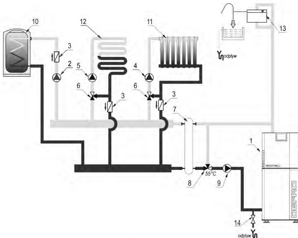
Rysunek 7. Uproszczony schemat instalacji grzewczej systemu otwartego.
