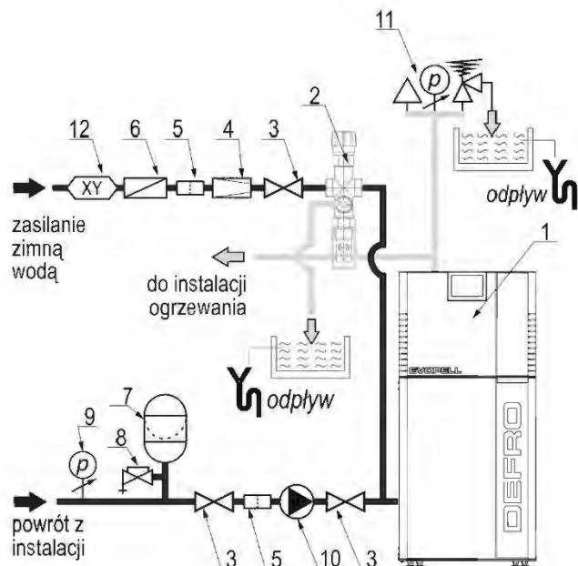
Rysunek 5. Przykładowy schemat zabezpieczeń kotła w układzie zamkniętym:
