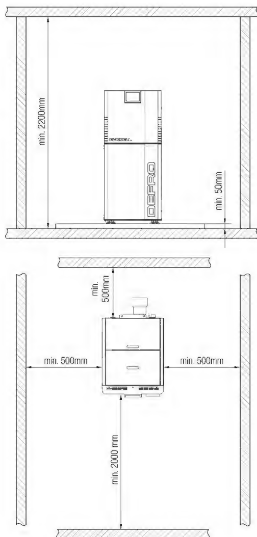
Rysunek 3. Ustawienie kotła w pomieszczeniu kotłowni.
