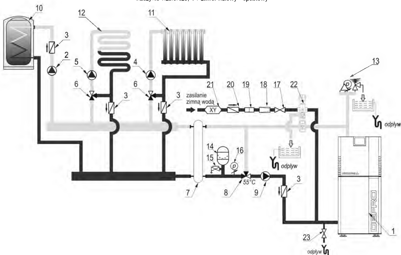
Rysunek 8. Uproszczony schemat instalacji grzewczej systemu zamkniętego.
